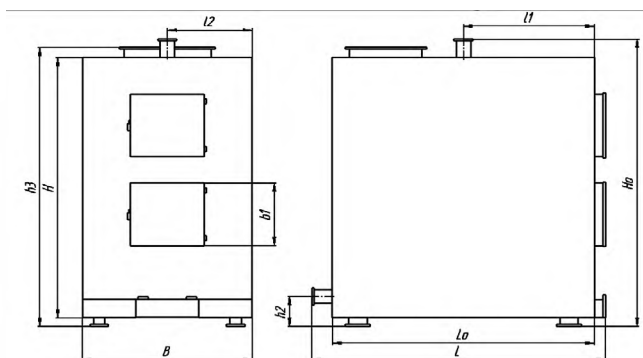
Рис. 1 — Чертёж Изделия
