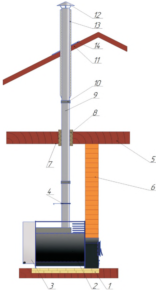
Рис. 3 - Рекомендуемое расположение банной печи с дымоходом.
