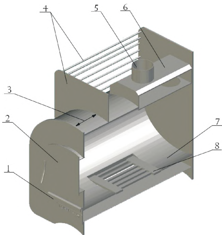
Рис. 2 - Схематичное изображение печи
